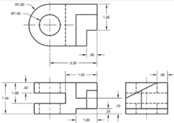
Belajar lukisan orthographic
